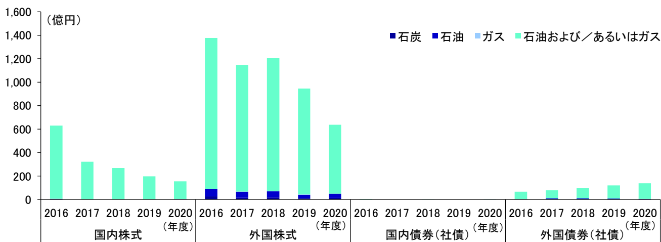
図表 1-33 化石燃料関連事業の設備投資総額
