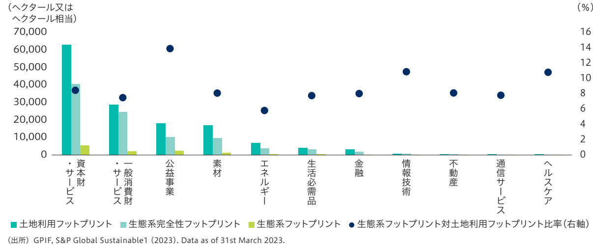
【図表8】外国株式のセクター別の自然への影響
