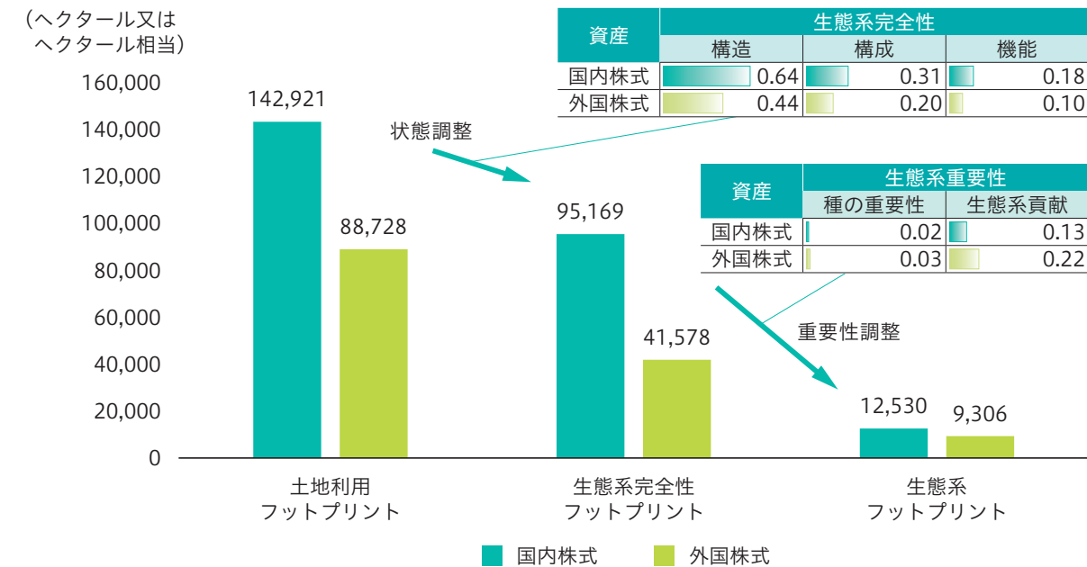
【図表6】国内株式と外国株式の自然への影響
