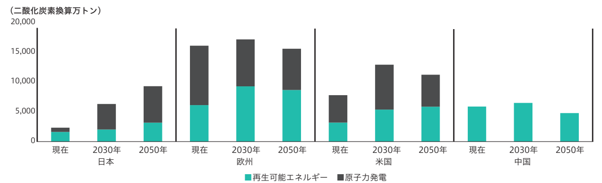
【図表5】発電事業の削減貢献量の地域毎の比較
